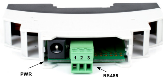
Abbildung 2: Pinbelegung BUS Auskoppler
