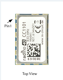
Module height: 3.6 ± 0.15 mm
