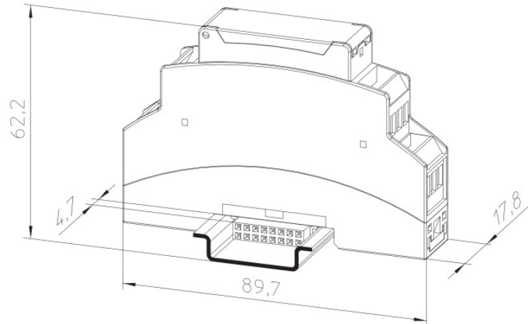
Abbildung 3: Maßzeichnung
