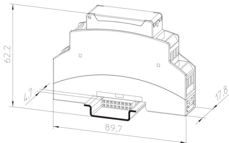
Abbildung 3: Maßzeichnung
